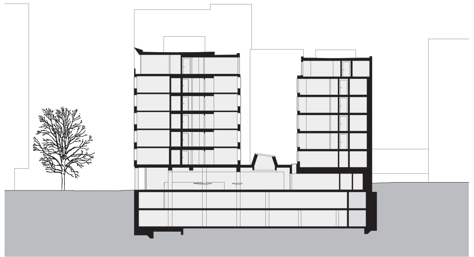
Schnitt: Das Erdgeschoss verbindet Vorder- und Hinterhaus.
