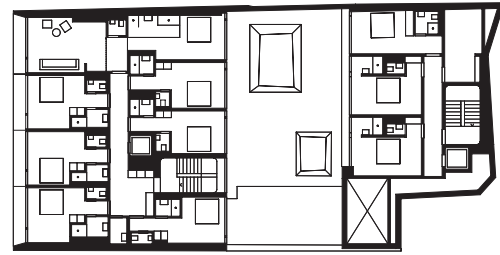
Das sechste Obergeschoss mit Attika-Aufbau.
